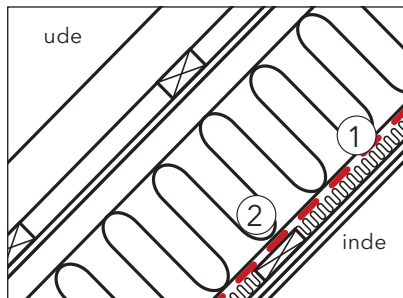
Principløsning - Skråvæg i stål.
