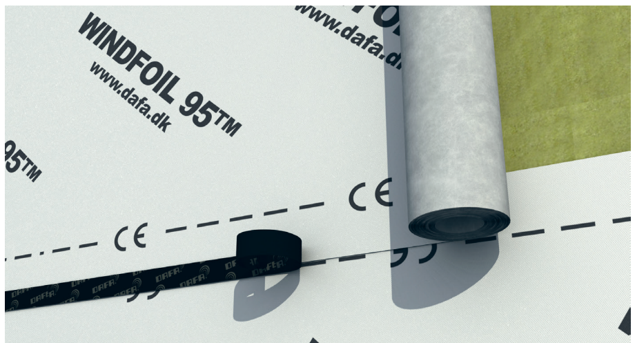
DAFA WindFoil 95 som vindspærre monteres med 150 mm overlæg, og samlinger tapes med DAFA UV tape.
